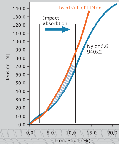
Tensile Strength
